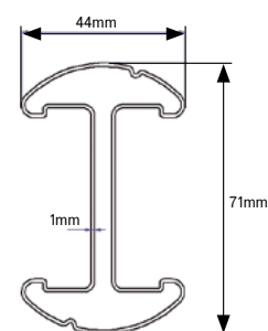
Vue de coupe du poteau EXPERT (260S)
